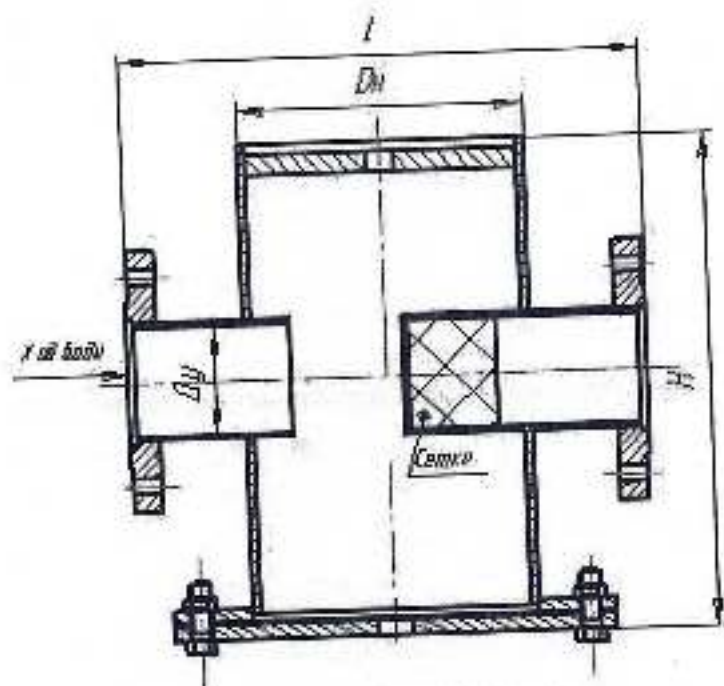
2 Исполнение фланцевое
